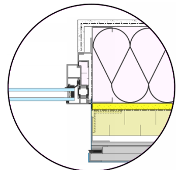
Jamb Detail
