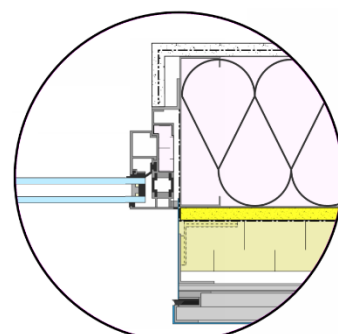
Jamb Detail
