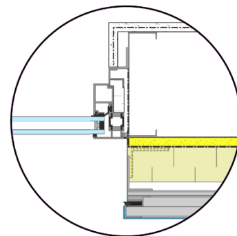
Jamb Detail
